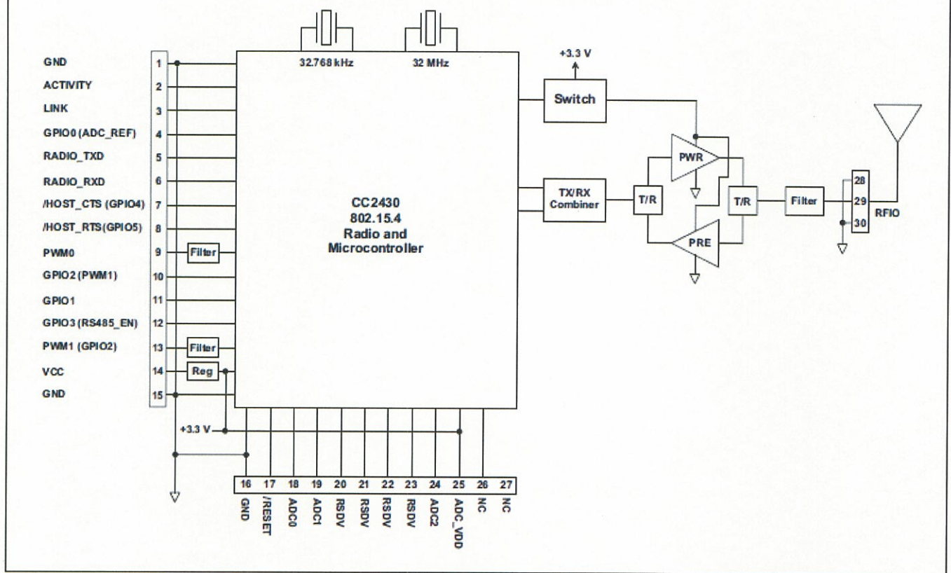
図1: LPR2430ERブロックダイアグラム
