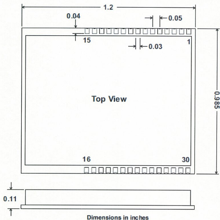
図2: LPR2430ERアウトライン及び実装寸法
